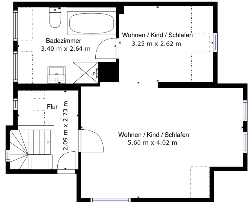
Dachgeschoss
